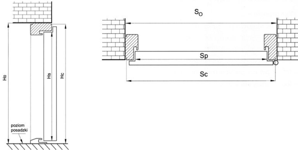
Wymiarowanie drzwi z ościeżnicą "11", "12", aluminiowo-kompozytowa oraz TERMO i TERMO PRESTIGE
