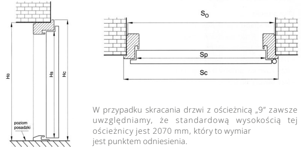
Wymiarowanie drzwi z ościeżnicą "9"
